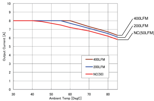
図 12 条件：Vin=12.0V, Vo=6.6V
