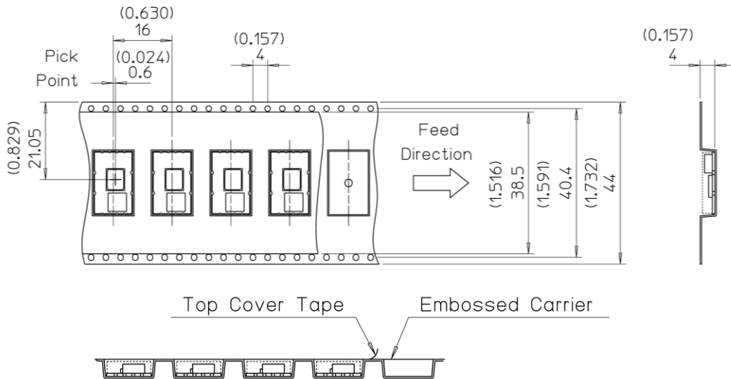
図 20 テープ寸法
