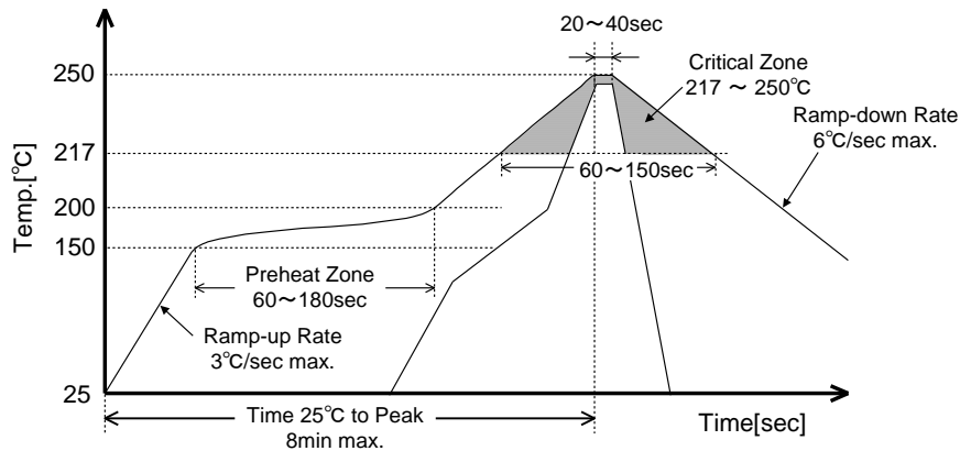
図 18 フロー温度プロファイル（鉛フリー）
