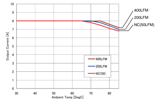
図 15 条件：Vin=12.0V, Vo=0.8V
