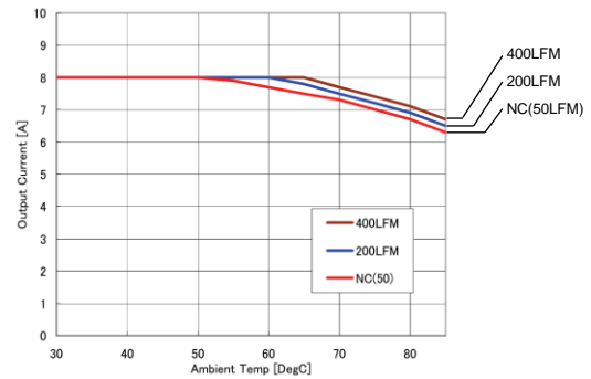
図 13 条件：Vin=12.0V, Vo=3.3V
