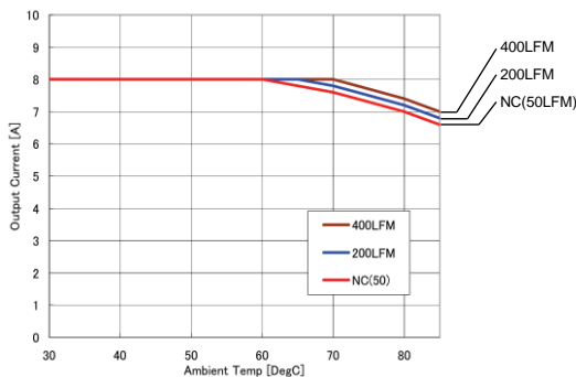
図 14 条件：Vin=12.0V, Vo=1.8V
