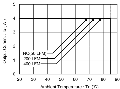
図 13 条件：Vin=12.0V, Vo=0.8-6.6V
