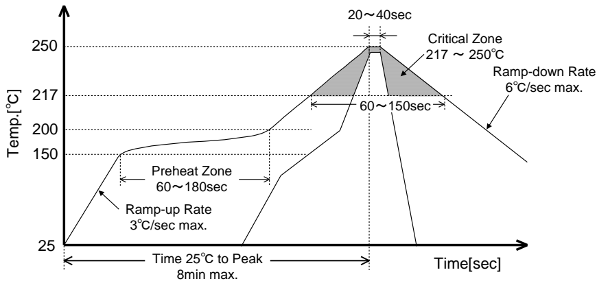
図 16 フロー温度プロファイル（鉛フリー）
