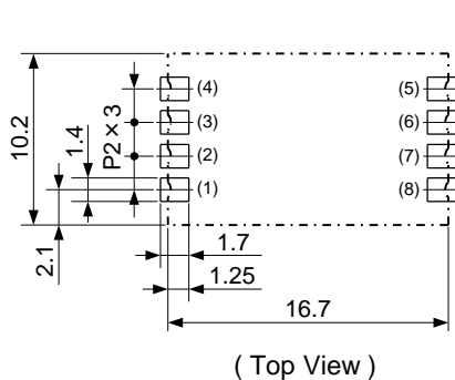
図 4 パッド (9) を接続しない場合
