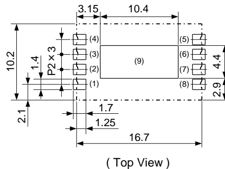
図 5 パッド (9) を接続する場合
