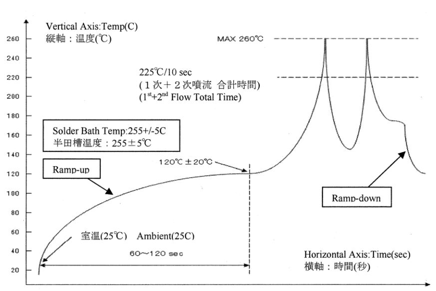
図 15 フロー温度プロファイル（鉛フリー）
