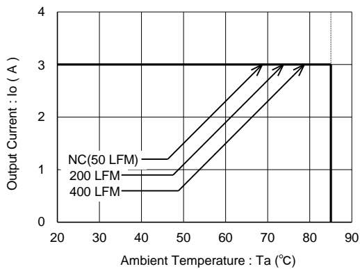
図 12 条件 : V_{in}=12.0V , V_o=0.8-6.6V (参考データ)
