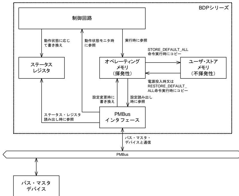
デジタル制御概念図
