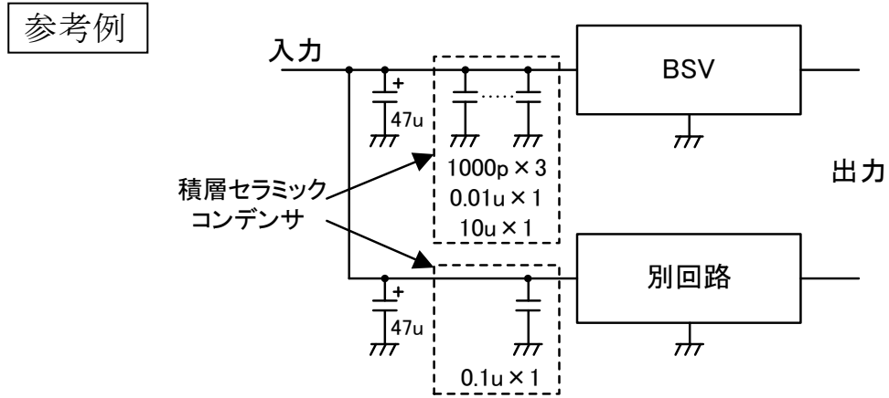
[ BSV 入力側積層セラミックコンデンサの構成と配置 ]
