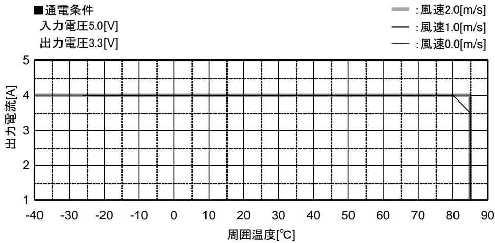
BSV-3.3S4R0M 温度ディレーティング
