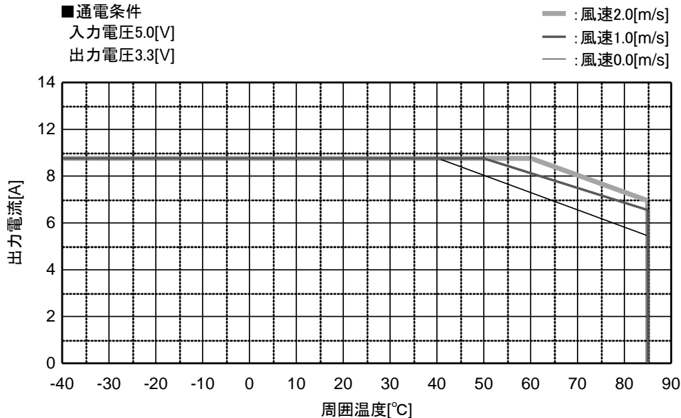
BSV-3.3S9R5M 温度ディレーティング
