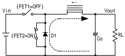
(b) toff時のメイン電流の流れ
