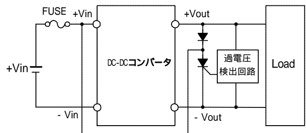
過電圧保護回路参考例
